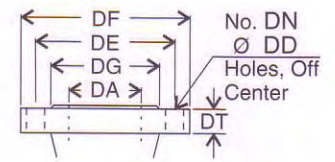
Discharge Flange Dimensions (JIS 10kgf/cm 2 )
